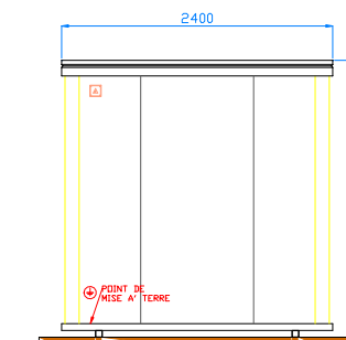
COTE' DROITE
